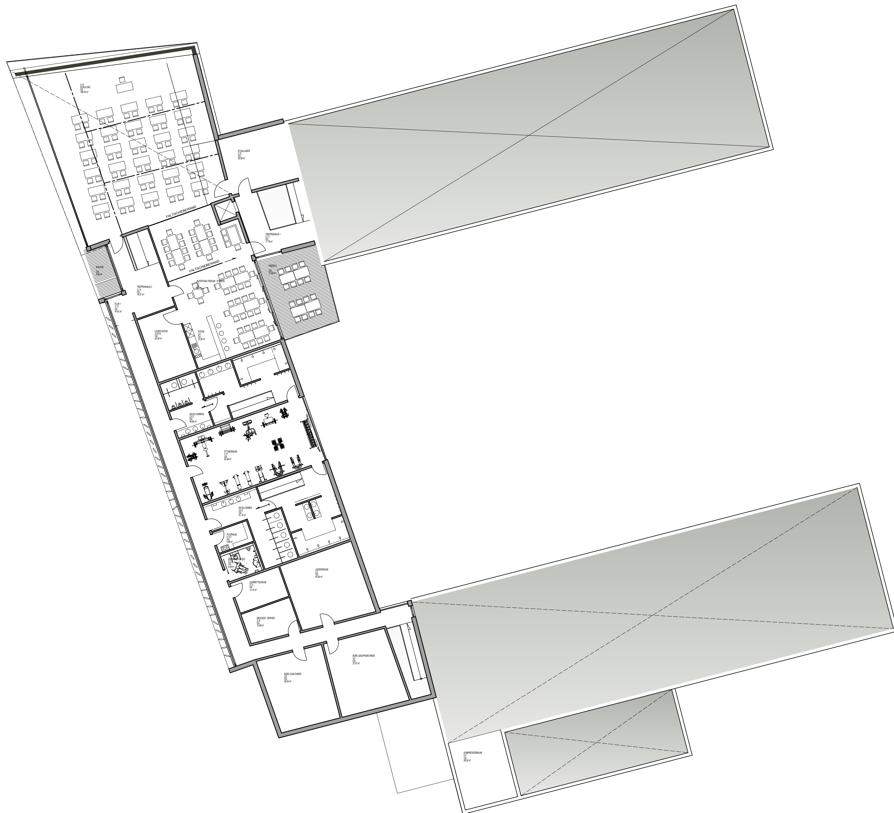
OBERGESCHOSS
