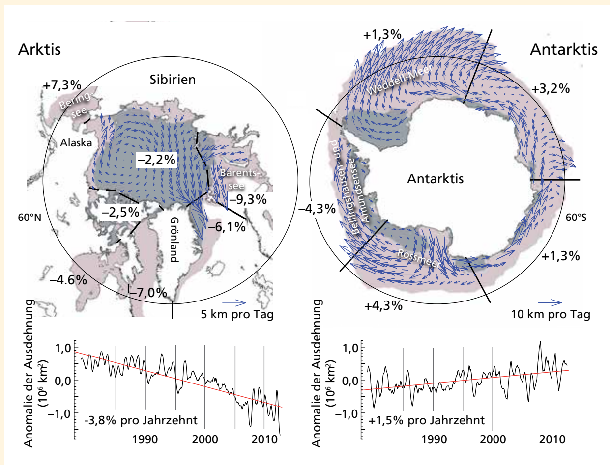
FAQ 4.1, Abbildung 1 | Mittleres Zirkulationsmuster von Meeris und die dekadischen Trends (%) der jährlichen Anomalien der Meereisausdehnung (d. h. nach Entfernung des Jahresgangs) in verschiedenen Regionen der Arktis und Antarktis. Pfeile zeigen die mittlere Richtung und Geschwindigkeit der Eisdrift an. Die mittlere Meereisbedeckung, beruhend auf Satellitenbeobachtungen, in maximaler (minimaler) Ausdehnung im Zeitraum von 1979 bis 2012 ist in Orange (Grau) schattiert.
