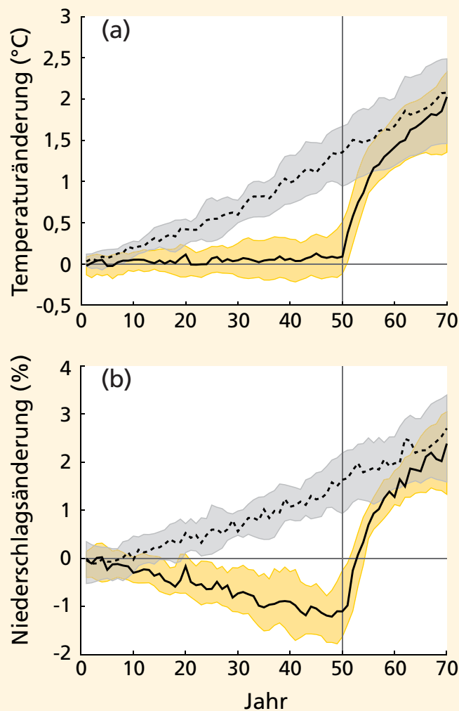
FAQ 7.3, Abbildung 2 | Änderung der global gemittelten (a) Erdoberflächentemperatur ( ^{\circ}\text{C} ) und (b) Niederschläge (%) in zwei idealisierten Experimenten. Die durchgezogenen Linien gelten für Simulationen, die „Solar Radiation Management“ (SRM) nutzen, um einen Anstieg der \text{CO}_2 -Konzentration von 1 % pro Jahr bis zum Jahr 50, in dem das SRM endet, auszugleichen. Die gestrichelten Linien gelten für Simulationen mit einem Anstieg der \text{CO}_2 -Konzentration von 1 % pro Jahr ohne SRM. Die gelben und grauen Flächen markieren den Bereich zwischen dem 25. und dem 75. Perzentil aus acht verschiedenen Modellen.
